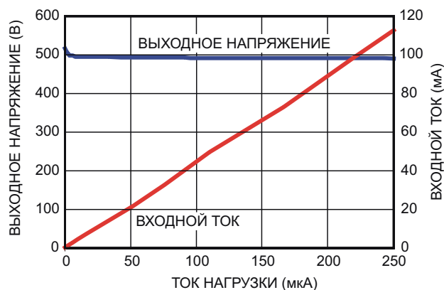
Рисунок 3. Зависимость выходного напряжения и входного тока от тока нагрузки.
