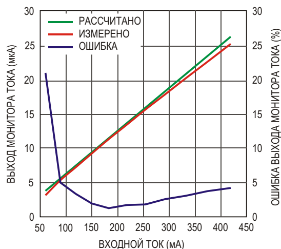
Рисунок 4. Зависимость сигнала монитора входного тока от тока входа.
