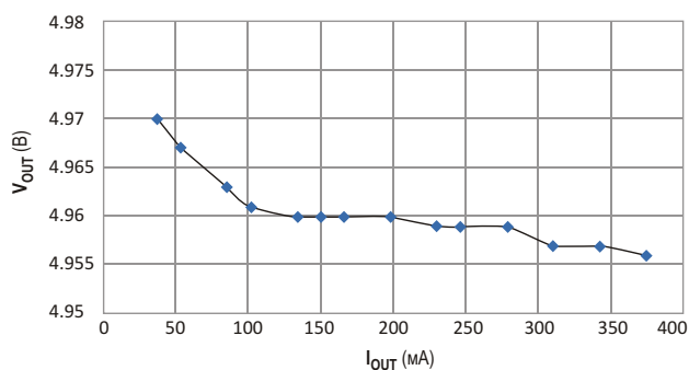
Рисунок 3. Во всем диапазоне токов нагрузки выходное напряжение изменяется менее чем на 14 мВ.
