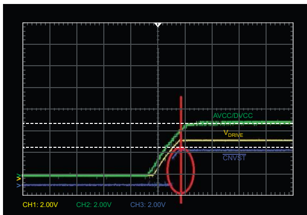
Рисунок 1. Подача высокого уровня на вход \overline{\text{CNVST}} во время установления напряжений питания может стать причиной неопределенного состояния АЦП.
