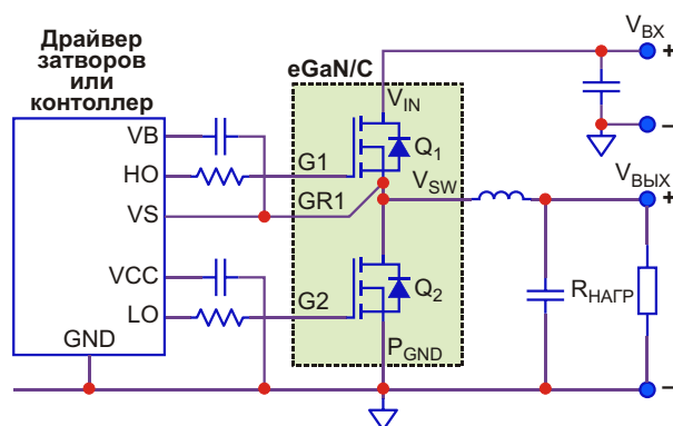
Типовая схема включения EPC2102/EPC2103.
