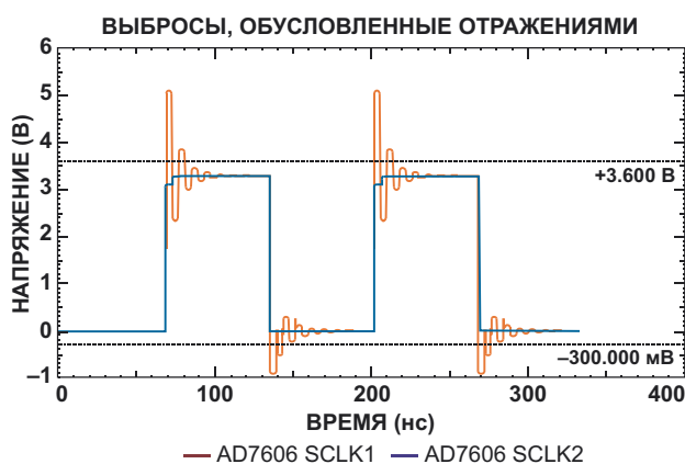
Рисунок 9. Результаты IBIS-моделирования выбросов на входе синхронизации AD7606.
