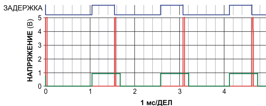
Рисунок 3. Результат регулировки задержки показан при той же установке длительности, как и на Рисунке 2. Верхняя линия (синяя) отображает задержку строба, нижняя (зеленая) – продолжительность импульса на базе Q 1 , а 5-вольтовая красная – тактовую частоту.
