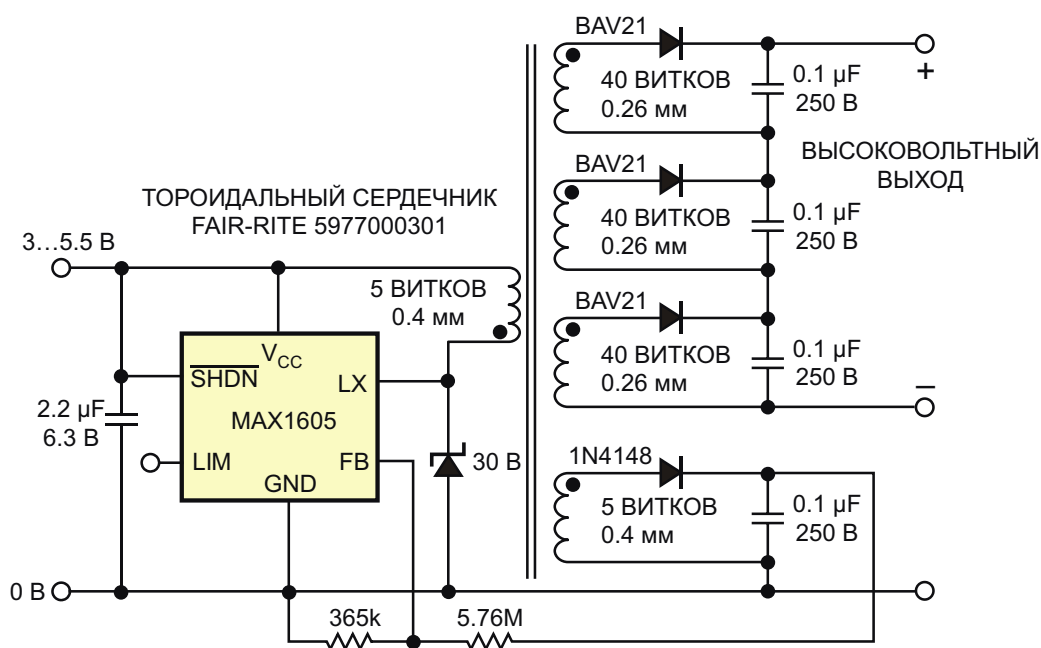
Рисунок 1. Используя сигнал обратной связи от низковольтной вторичной обмотки, этот высоковольтный источник питания с малым током покоя генерирует напряжение в 500 В.
