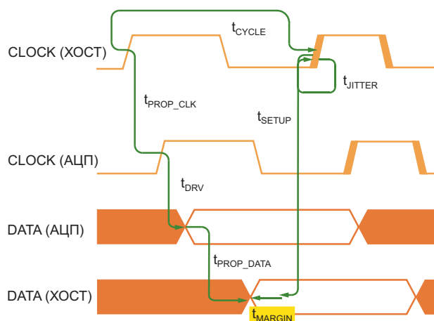
Рисунок 2. Запасы по времени установления и удержания.
