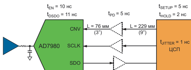
Рисунок 4. Цифровой интерфейс между ЦСП и микросхемой AD7980.
